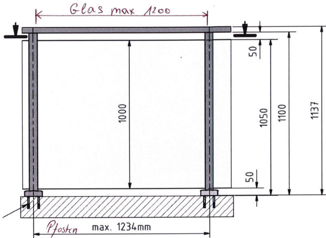
Abb. 1 Pfosten GOTU Top Handlauf
