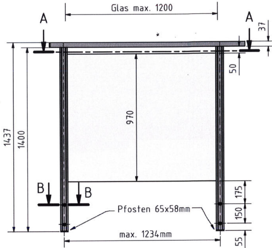
Abb. 4 Pfosten GOTU Side Handlauf
